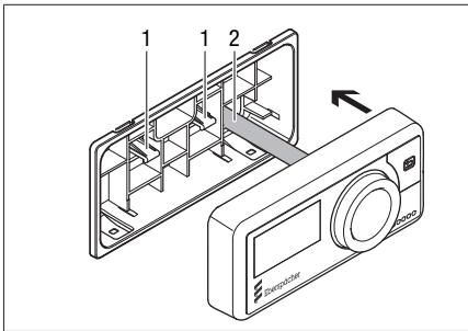
1 Halteclips 2 Anschlussleitung
